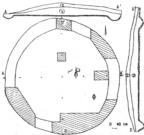
Рис. 6. Городище, с. Курганний некрополь III. Курган № 2/1995 р. План і перетини. За В. В. Приймаком.
