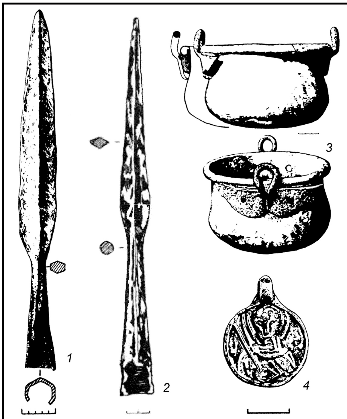
Рис. 5. Лохвиця-2. Знахідки із городища в ур. Високі Лазірки Окремі знахідки з пам'ятки. 1-2 – залізо, 3 – залізо, мідь; 4 – бронза. За: Ю. Моргуновим, 1996, О. Супруненьком, І. Кулатовою, О. Тітковим, К. Мироненком, 2003.
